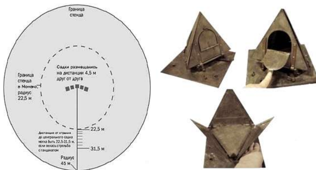
Схема устройства площадки стенда для садочной стрельбы и садки для запуска птицы.
